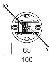
SNODO CON ADATTATORE PER UNITÀ RIFLETTENTE (a richiesta)
