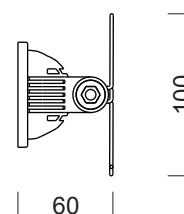
SNODO CON ADATTATORE PER UNITÀ RIFLETTENTE (a richiesta)
