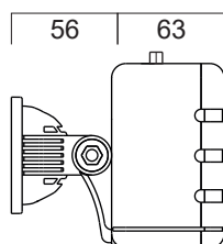
VISTA LATERALE (snodo a richiesta)
